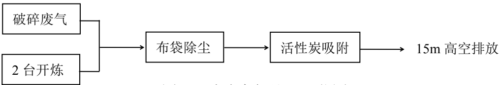
图 4-2 破碎废气处理工艺图
