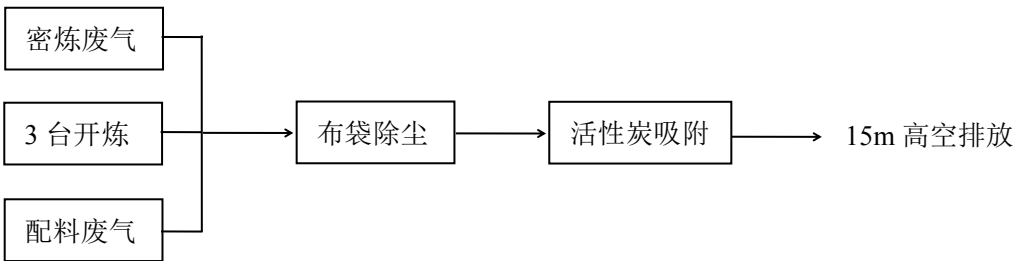
图 4-1 炼胶废气处理工艺图
