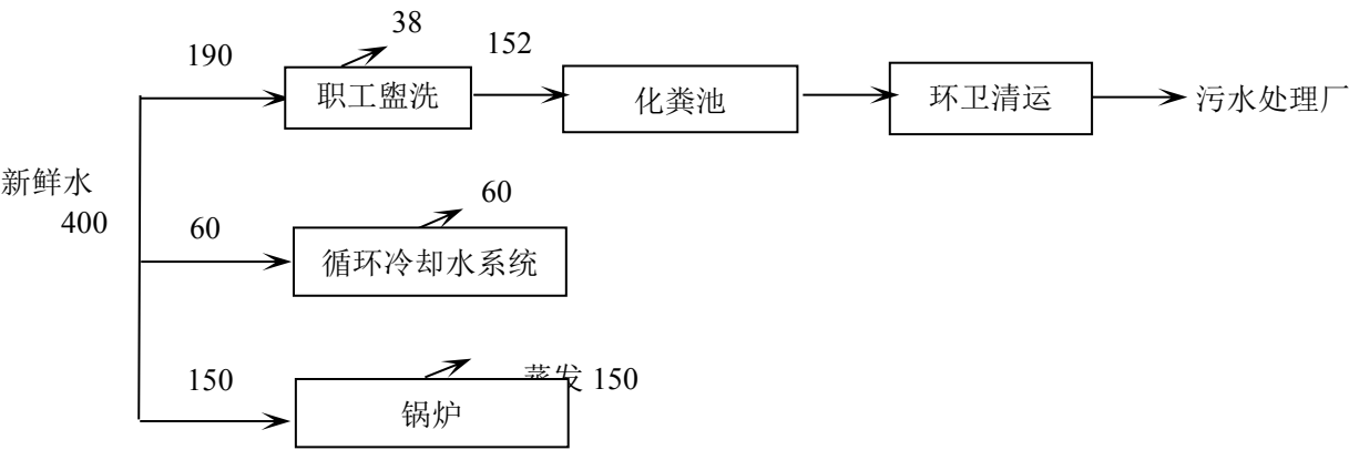
图 3-1 厂区实际用水平衡图 单位：t/a
