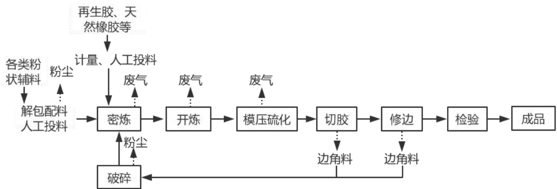
图 3-2 工艺流程及排污节点
