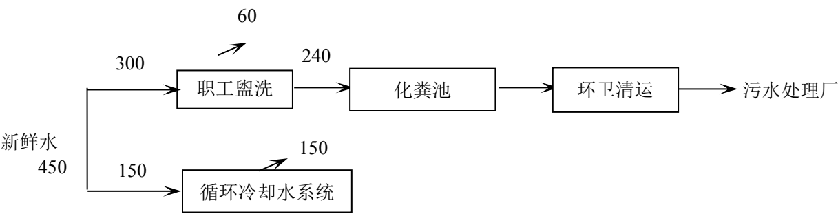
图 3-1 厂区实际用水平衡图 单位：t/a
