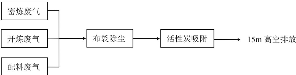
图 4-1 炼胶废气处理工艺图
