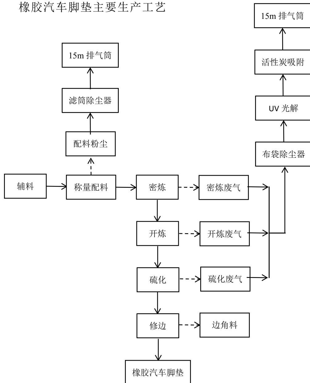
图 3-2 项目橡胶汽车脚垫生产工艺流程图
