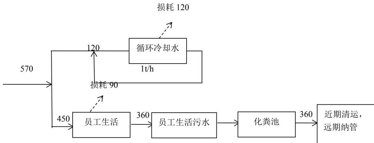
图 3-1 项目水平衡图 (单位: t/a)
