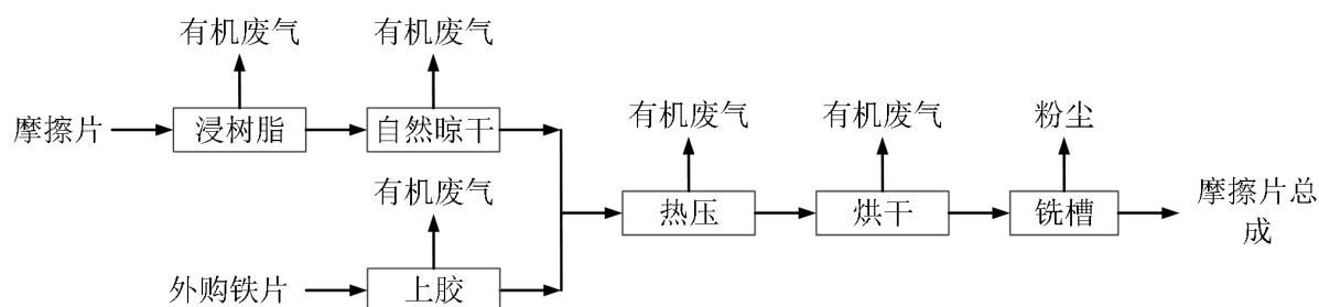
图2-8 摩擦总成生产工艺流程图
