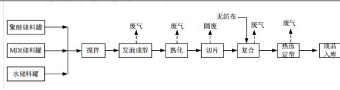
图2-3 汽车隔音隔热内饰件生产工艺流程图
